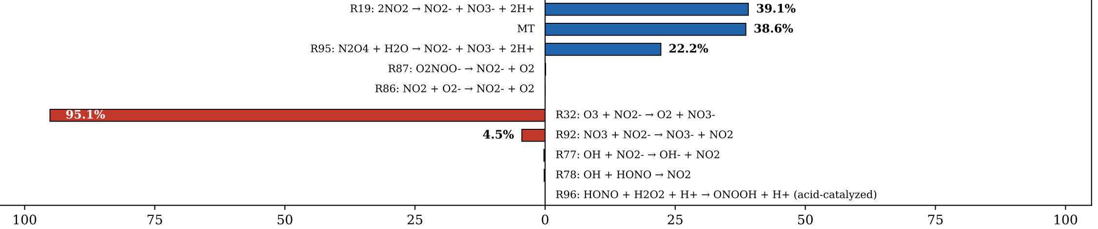
(d) H 2 O 2 (Σsrc = 2.77e-08 M/s)
